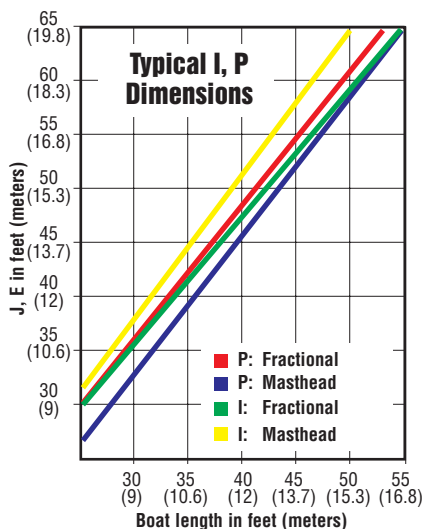
Rig Dimensions
